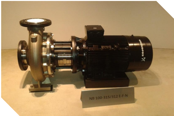
Pump NB - 100-315
