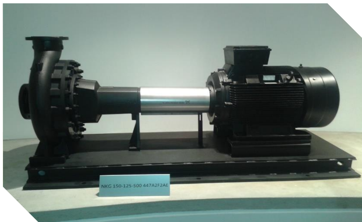
Центрифугална Пумпа NKG - 150-125
