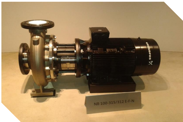
Пумпа NB - 100-315
