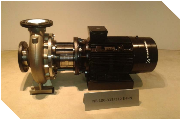
Насос NB - 100-315
